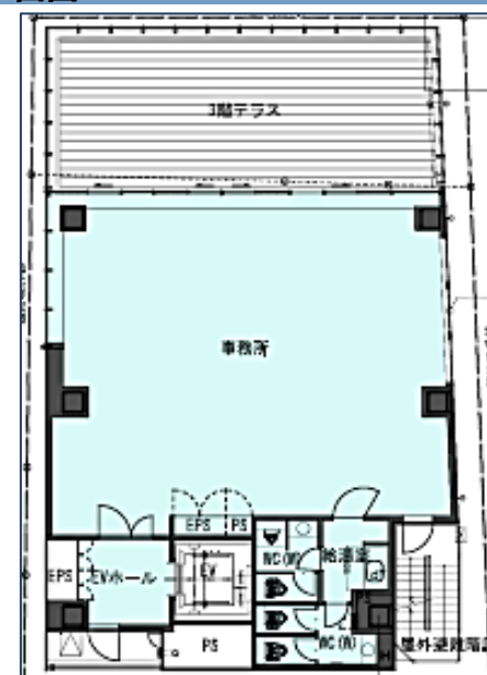
3階平面図
